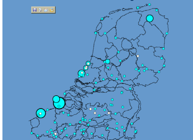
Alle Koperwiek in periode 7 oktober 2004 t/m 12 oktober 2004. Totaal 380088 vogels.
